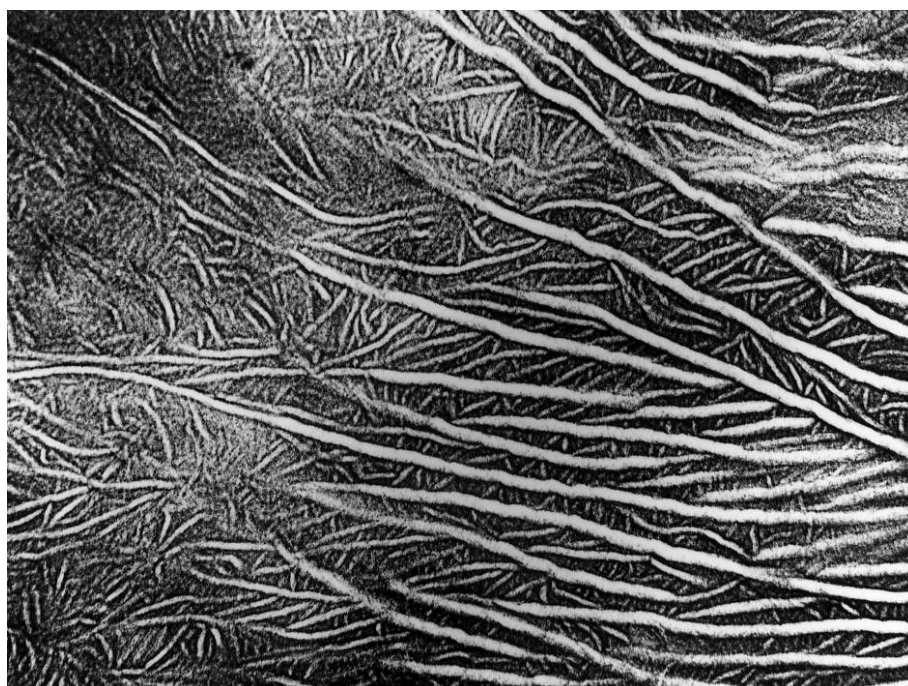
HDPE/L-LDPEブレンド
