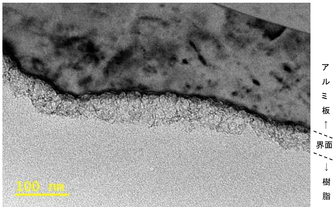
PPS樹脂/アルミ板接合界面
